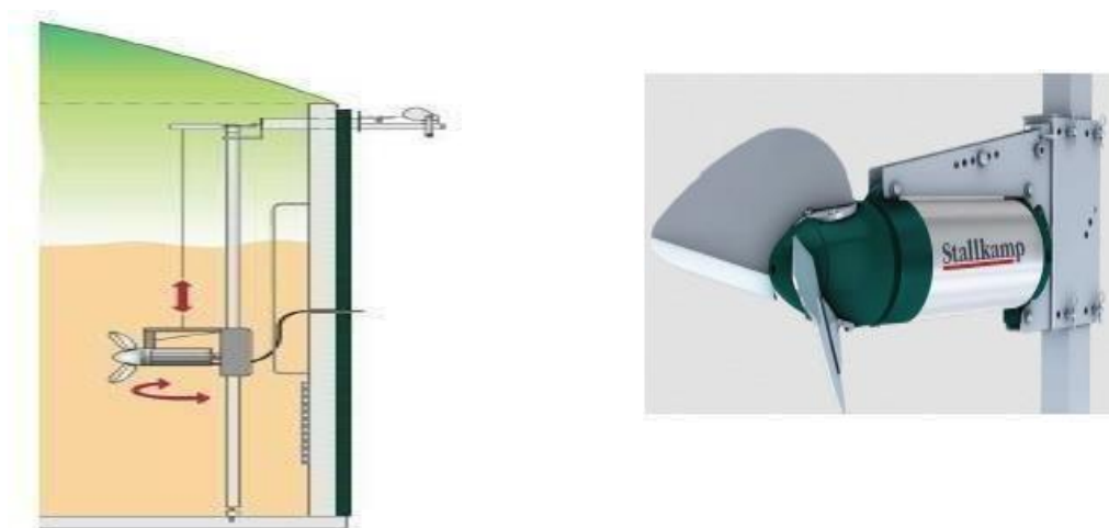
डाइजेस्टर के अंदर सबमर्सिबल मिक्सर
