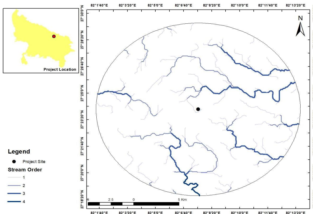
चित्र 2-3 बलरामपुर स्थल के निकट धारा नेटवर्क
